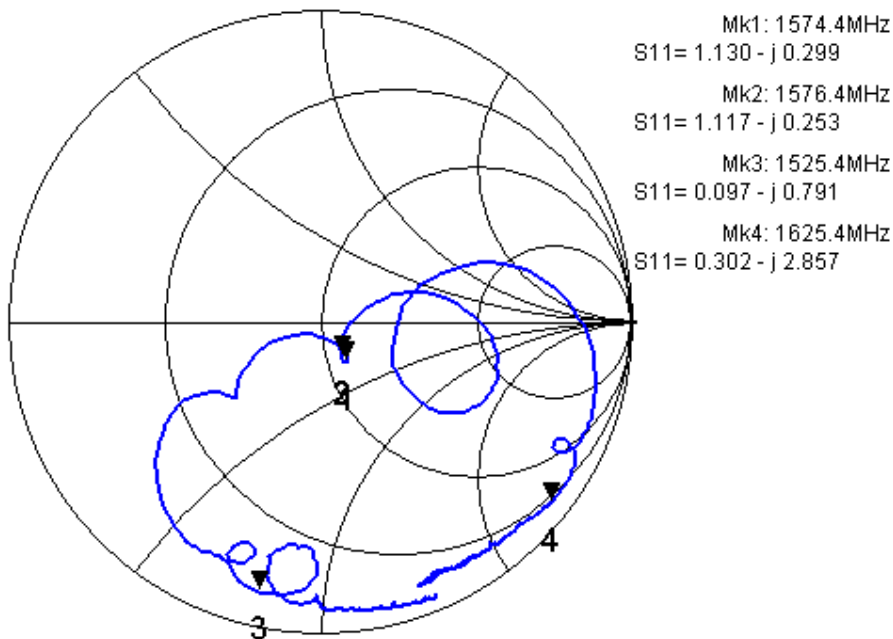
Fig.5 Input Impedance
