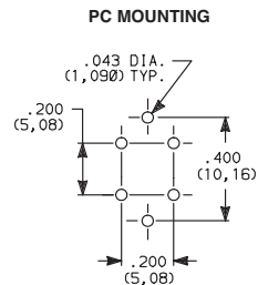
EP21SD1V3BE DPST
