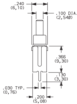
V31 SNAP-IN
