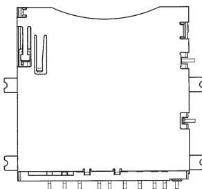
スプリングイジェクト ノーマルタイプ H=2.8MM SPRING EJECT NORMAL TYPE H=2.8MM
