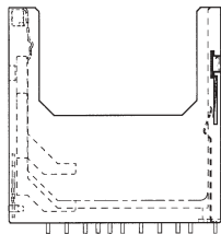
スプリングイジェクト ノーマルタイプ SPRING EJECT NORMAL TYPE
