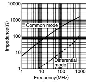
ACM2520-102-2P
