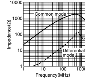
ACM3225-102-2P
