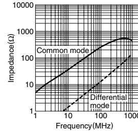
ACM3225-271-2P
