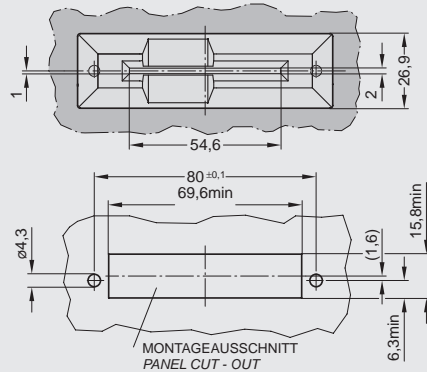
MONTAGEBLECH C702 G51 012 E2:
