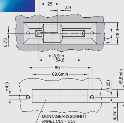
MONTAGEBLECH C702 G51 012 E2:
