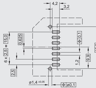
LEITERPLATTEN - BESTÜCKUNG PCB - LAYOUT
