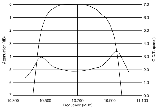
SFECF10M7DA0001-R0
