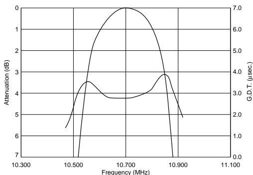
SFECF10M7FA00-R0/SFECF10M7FF00-R0
