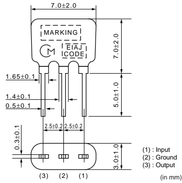
SFVLF10M7LF00-B0
