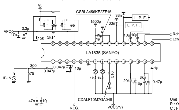
CDALF10M7GA048-B0
