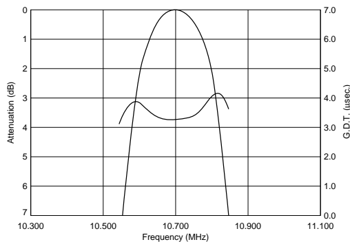
SFECF10M7GA00-R0/SFECF10M7GF00-R0
