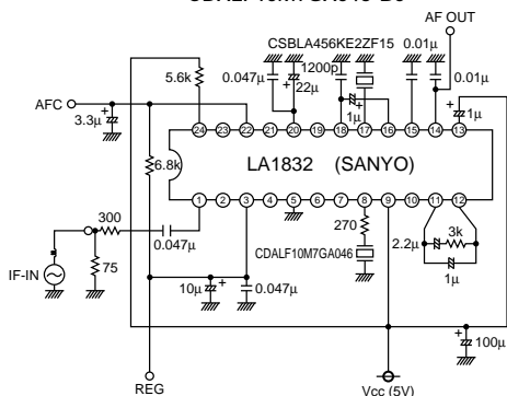
CDALF10M7GA046-B0
