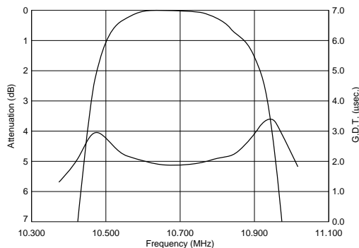
SFECF10M7DF00-R0
