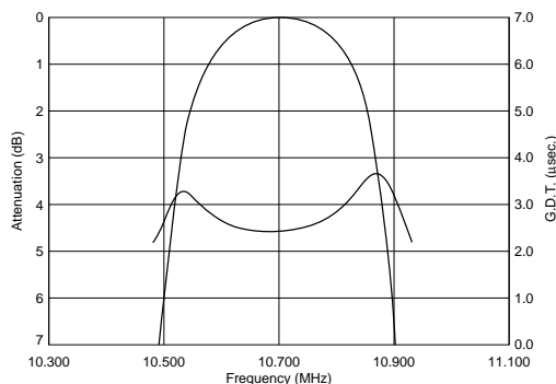
SFECF10M7EA00-R0
