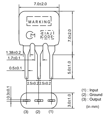
SFELF10M7KAH0-B0
