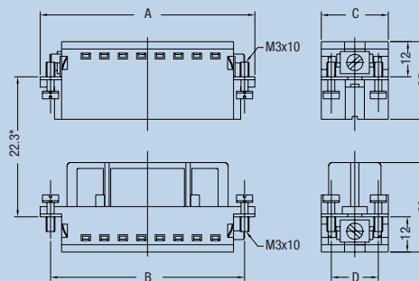
*Abstand für sichere Kontaktgabe 24 mm
