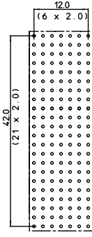
LAY-OUT P.C.B. -HOLES
