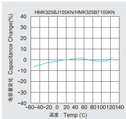
电容量—温度特性 Temperature characteristics
