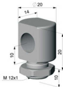
Montagebolzen mit M12x1-Gewinde
