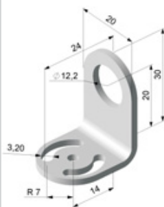
Montagewinkel, fest
