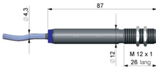
Abmessungen CS
