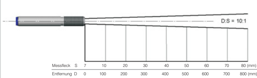
10:1 Optik
