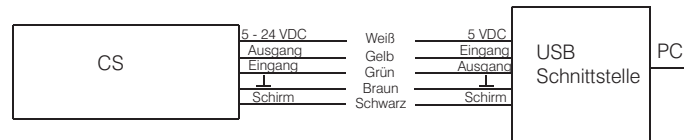
Schnittstellendiagramm CS/USB programmierbare Schnittstelle
