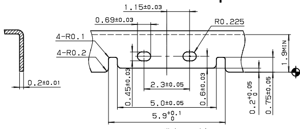
シールドケース形状 (S=10/1) SHIELDING CASE FORM
