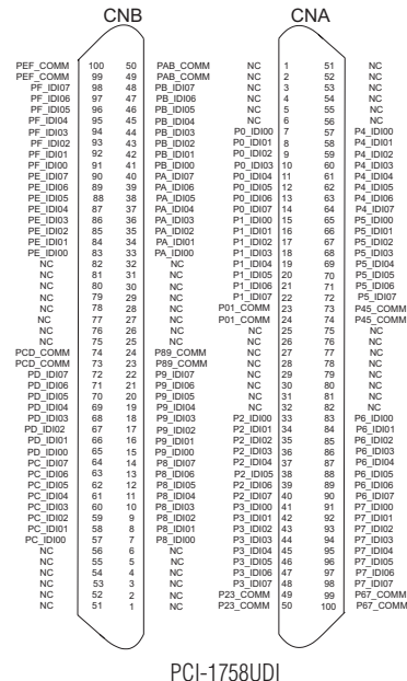
PCI-1758UDI
