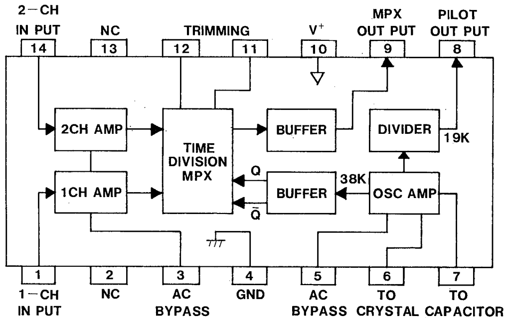
NJM2035D NJM2035M
