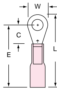
MH18-8R/L Stud Size: 8 Wire Range: 22-18
