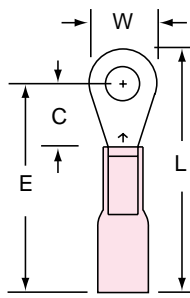
MH18-6R/L Stud Size: 6 Wire Range: 22-18
