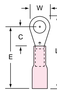
MH18-10R/L Stud Size: 10 Wire Range: 22-18
