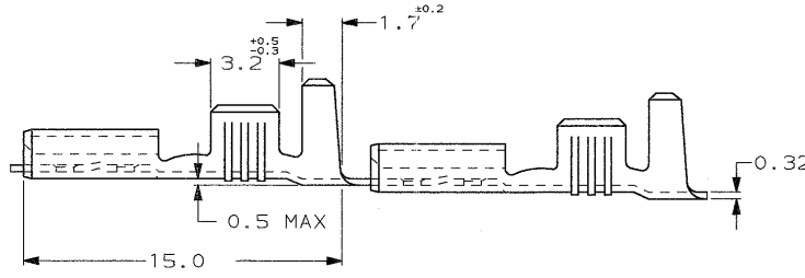
SEZIONE B-B (SECTION B-B)
