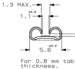
SEZIONE A-A (SECTION A-A)
