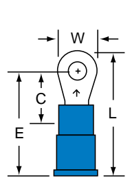
MV14-4R/S Stud Size: 4 Wire Range: 16-14
