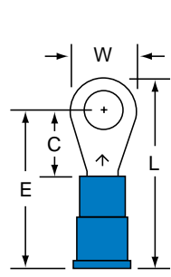
MV14-10R/L Stud Size: 10 Wire Range: 16-14
