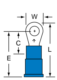
MV14-6R/S Stud Size: 6 Wire Range: 16-14
