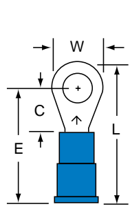
MV14-10R Stud Size: 10 Wire Range: 16-14
