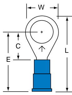
MV14-516R/S Stud Size: 5/16 Wire Range: 16-14
