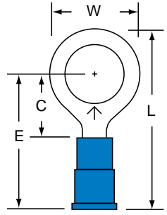
MV14-38R Stud Size: 3/8 Wire Range: 16-14
