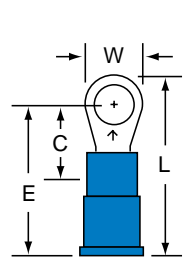
MV14-8R/S Stud Size: 8 Wire Range: 16-14
