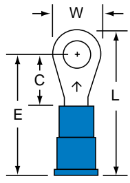
MV14-8R/L Stud Size: 8 Wire Range: 16-14
