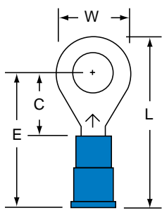
MV14-14R/S Stud Size: 1/4 Wire Range: 16-14
