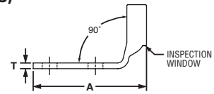
90° ANGLE TONGUE (Fig. 3)
