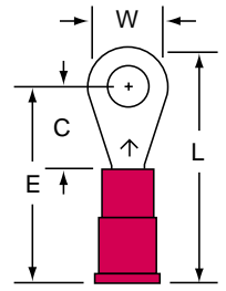
MVU18-8R/L Stud Size: 8 Wire Range: 22-18
