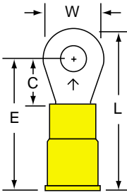
MVU10-8R Stud Size: 8 Wire Range: 12-10
