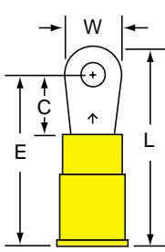
MVU10-4R/S Stud Size: 4 Wire Range: 12-10
