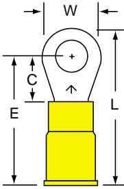
MVU10-10R Stud Size: 10 Wire Range: 12-10
