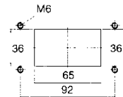
Montageausschnitt/Panel cut-out
