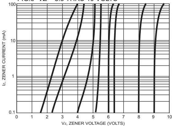
FIG.5- V_Z = 3.3 THRU 10 VOLTS
