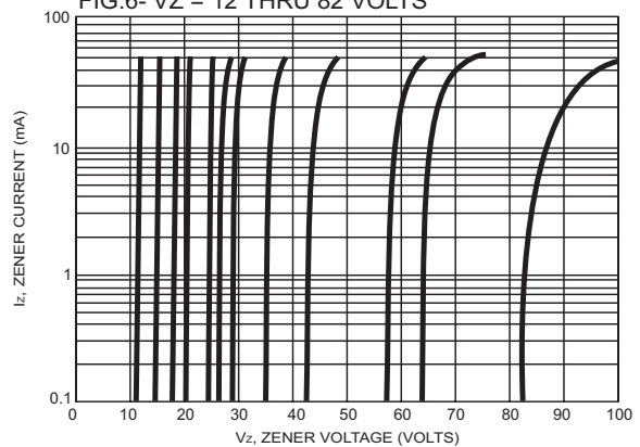
FIG.6- V_Z = 12 THRU 82 VOLTS
