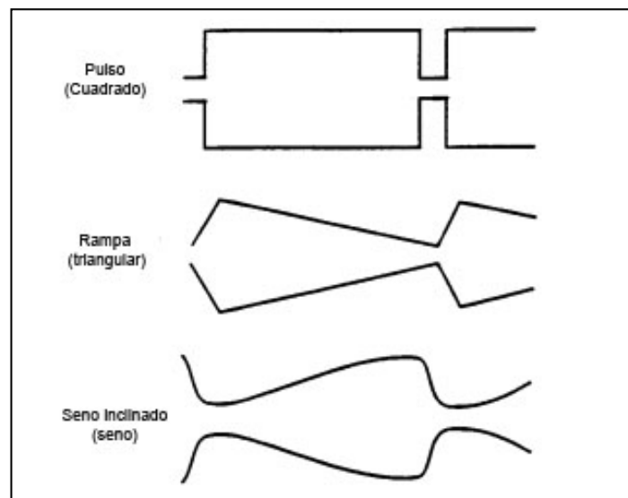
Figura 4 Efectos de variación de simetría
