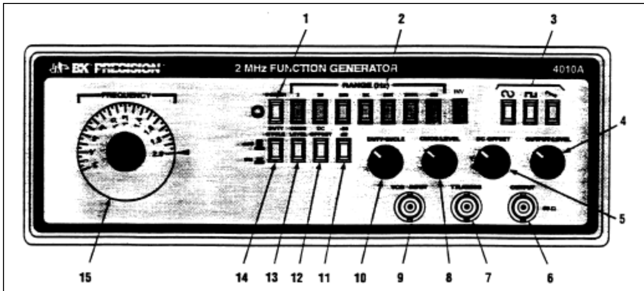
Figura 1. Panel frontal del modelo 4010A
