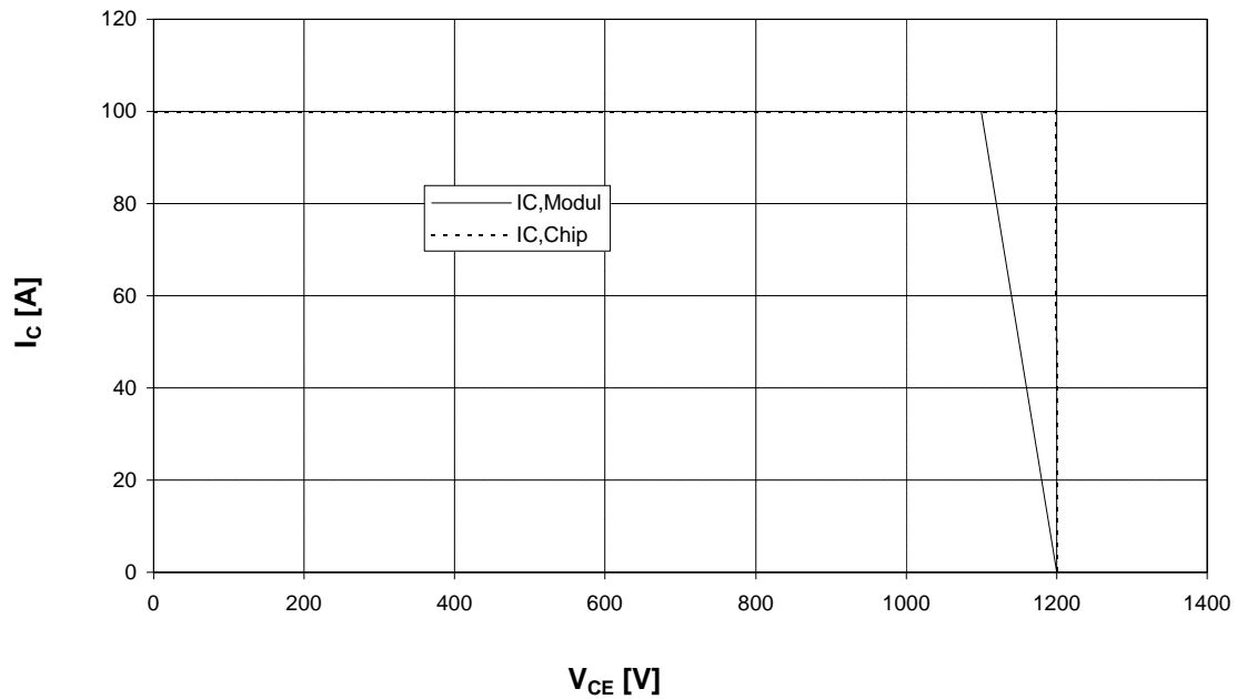
Sicherer Arbeitsbereich Wechslr. (RBSOA) I_C = f(V_{CE}) Reverse bias safe operating area Inverter (RBSOA) T_{vj} = 125^\circ\text{C} , V_{GE} = \pm 15\text{V} , R_G = 150\text{hm}
