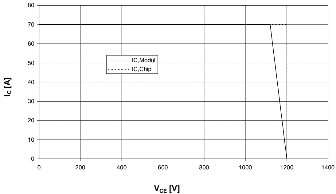
Sicherer Arbeitsbereich Wechselr. (RBSOA) I_C = f(V_{CE}) Reverse bias safe operating area Inverter (RBSOA) T_{vi} = 125^\circ\text{C} , V_{GE} = \pm 15\text{V} , R_G = 22\ \Omega
