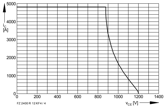
Bild / Fig. 4 Rückwärts-Arbeitsbereich / Reverse biased safe operating area T_{vj} = 125^\circ\text{C} V_{LF} = V_{LR} = 15 \text{ V} R_C = 0,47 \Omega
