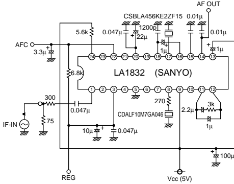
CDALF10M7GA046-B0
