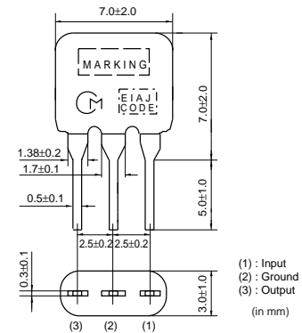
SFELF10M7DF00-B0
