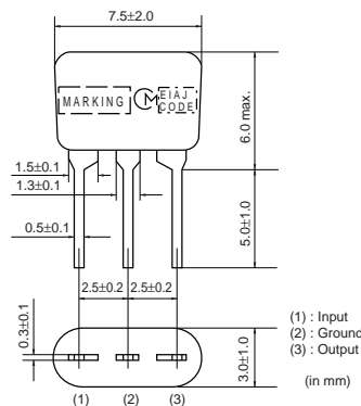
SFELG10M7GA00-B0
