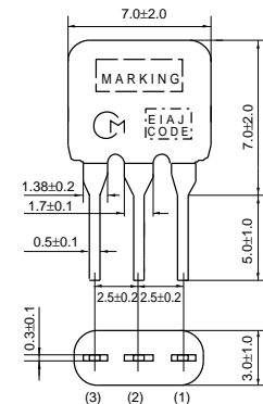
SFELF10M7HAA0-B0
