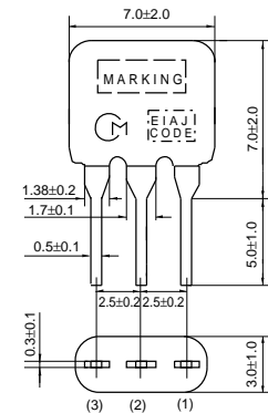
SFELF10M7FAA0-B0
