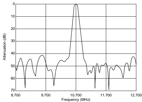
SFELF10M7KAH0-B0
