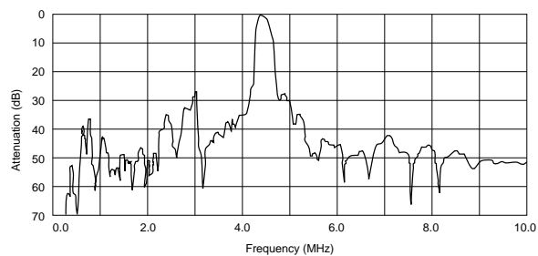
SFSKA4M50CF00-R1
