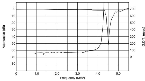
TPSKA4M50B00-R1
