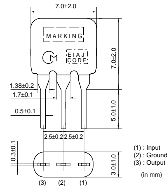
SFELF10M7DF00-B0
