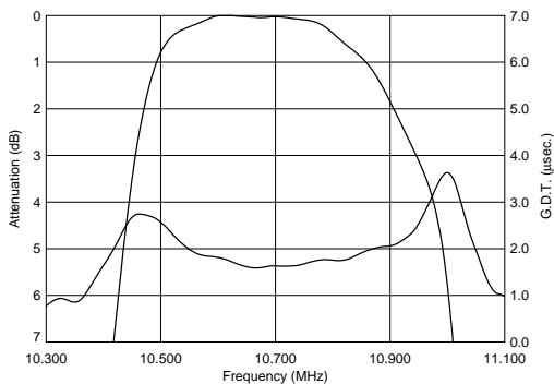
SFECF10M7CQ00-R0
