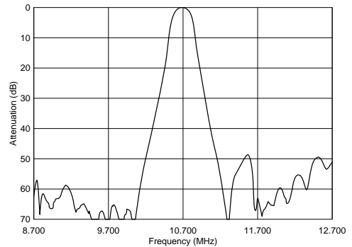
SFELG10M7GA00-B0
