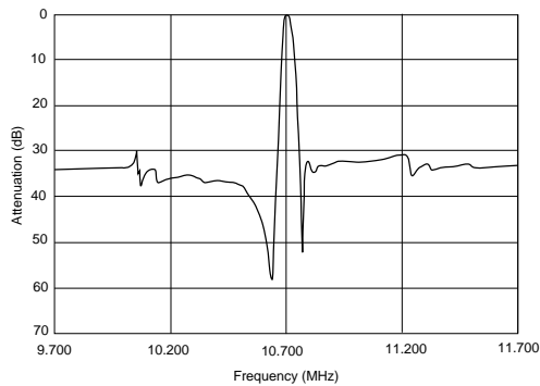
SFKLF10M7NL00-B0
