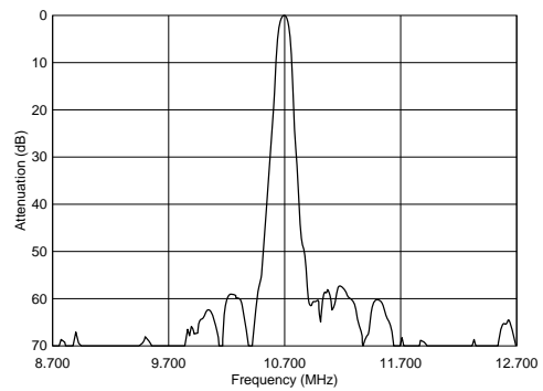
SFVLF10M7LF00-B0
