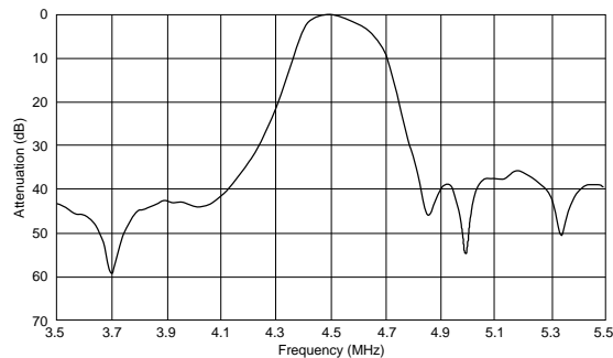
SFSRA4M50CF00-B0
