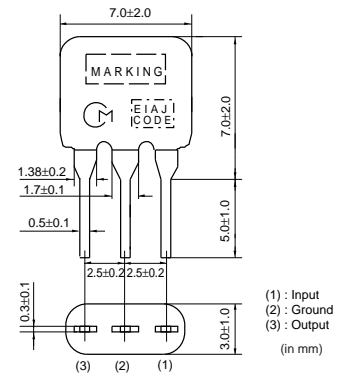
SFELF10M7KAH0-B0
