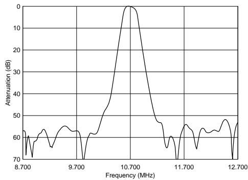
SFELF10M7GA00-B0
