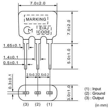
SFVLF10M7LF00-B0
