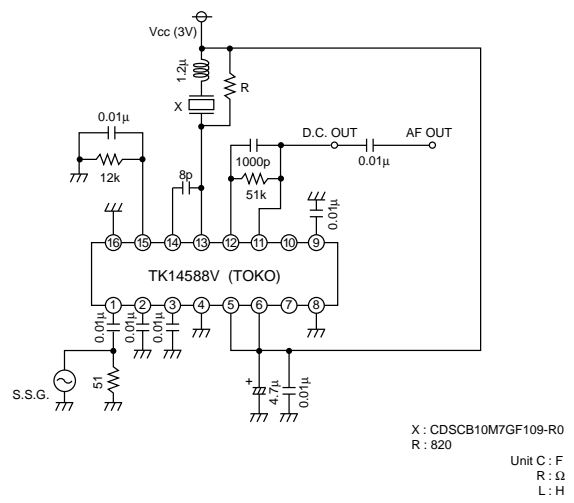
CDSCB10M7GF109-R0
