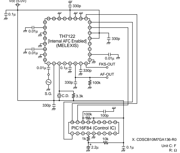
CDSCB10M7GA136-R0
