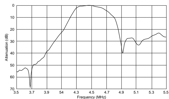
SFSRA4M50EF00-B0
