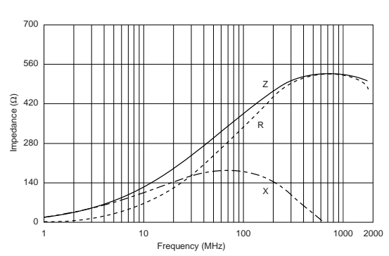
BLM18EG391TN1
