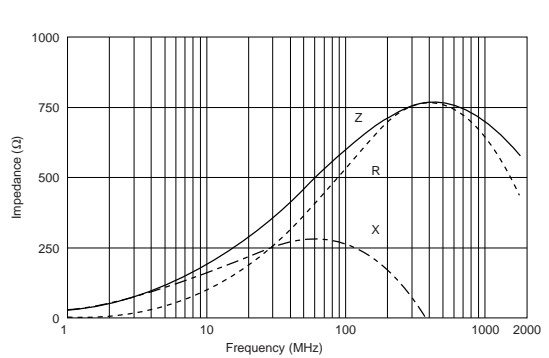
BLM18EG601SN1
