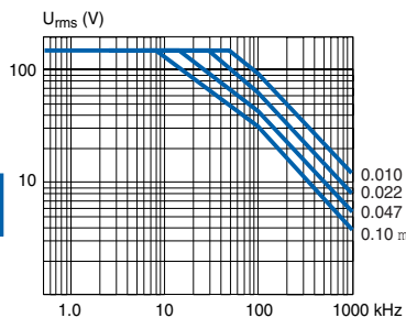
SMR5 250/160
