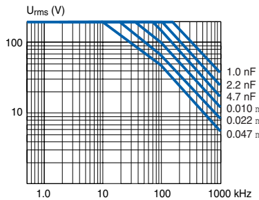
SMR5 400/200
