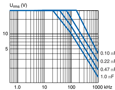
SMR5 50/30
