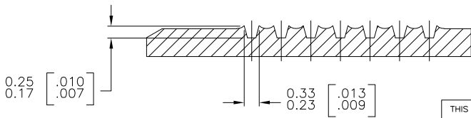
SECTION A-A SCALE 20:1
