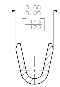
SECTION A-A SCALE 10:1
