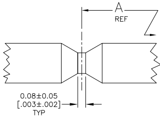
DETAIL W 30:1
