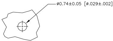
DETAIL W 30:1
