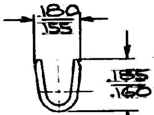
SECT A-A
