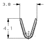
SEZIONE B-B (SECTION B-B)
