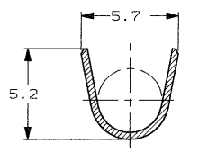
SEZIONE A-A (SECTION A-A)
