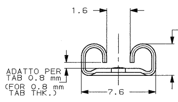
SEZIONE A-A (SECTION A-A)
