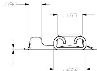
VIEW A-A
