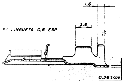
SEÇÃO "AA"
