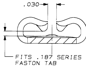
SECTION A-A SCALE 10:1
