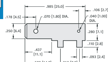
.250 (6.4) TAB
