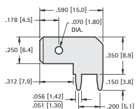
.250 (6.4) TAB
