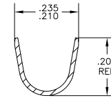
SECTION D-D
