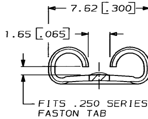
VIEW A-A
