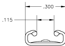
VIEW A-A
