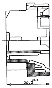
断面 A-A (SECT. A-A)
