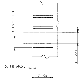
DETAIL C (SCALE: 10-1)
