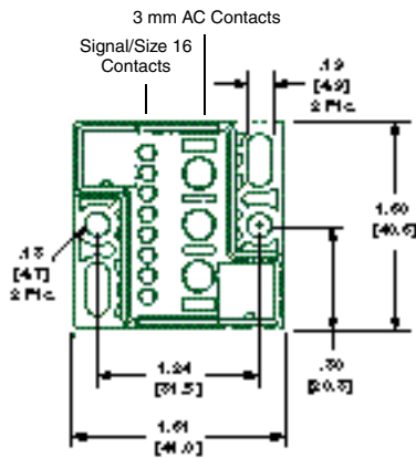
Receptacle 194279-1
