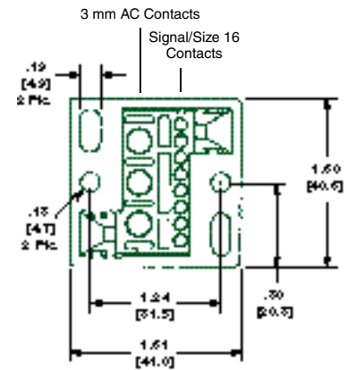
Plug 194278-1
